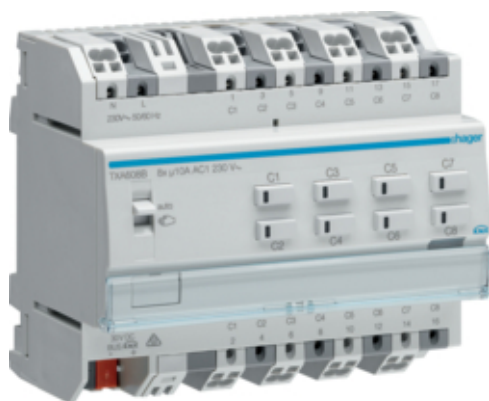
Mod. 8 sorties 10A/230V~ /NE
