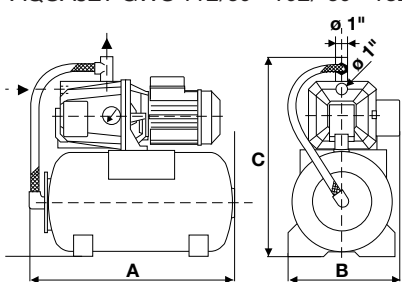
AQUAJET GWS 112/60 - 102/60 - 132/100
